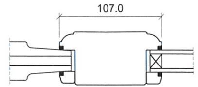
Lodret tapstykke
