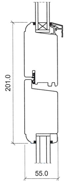
Midtersamling halvdør
