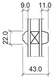
Pålagte sprosser
