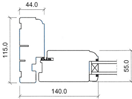
Sidekarm
