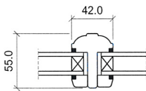
Lodret sprosse
