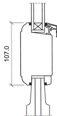
Vandret tapstykke
