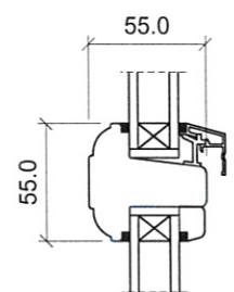
Vandret sprosse
