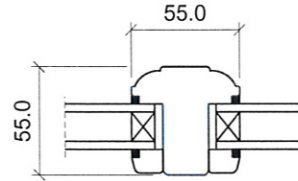
Lodret sprosse
