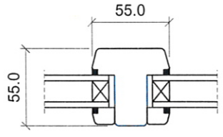
Lodret sprosse
