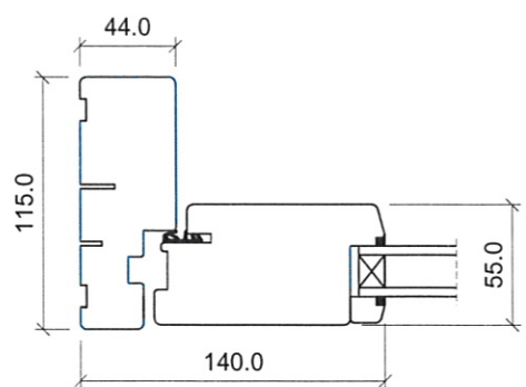
Sidekarm
