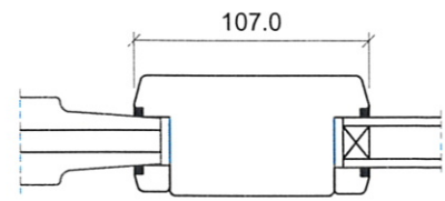
Lodret tapstykke
