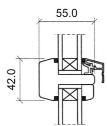
Vandret sprosse
