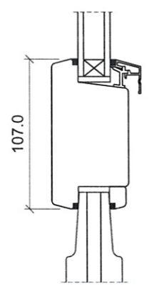
Vandret tapstykke
