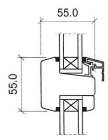
Vandret sprosse
