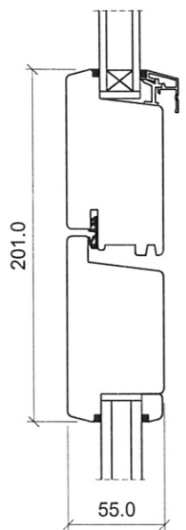
Midtersamling halvdør
