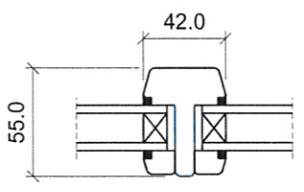
Lodret sprosse
