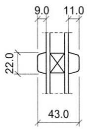
Pålagte sprosser
